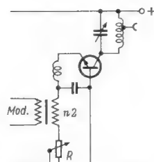
Bild 7. Emitterschaltung bei Basisschaltung der Endstufe
