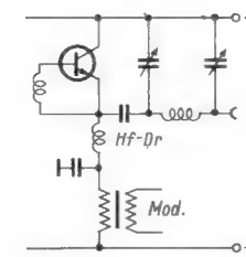
Bild 8. Emitterschaltung bei Emitterschaltung und geerdetem Kollektor
