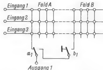
Bild 5. Umschaltbares Kreuzschaltfeld, für eine Tonleitung gezeichnet; die Stellung Feld A entspricht der mechanischen Ruhestellung
