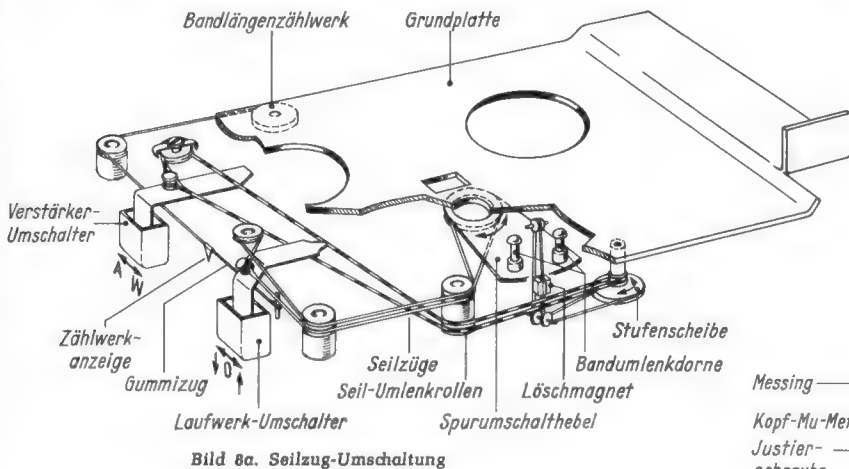
Bild 8a. Seilzug-Umschaltung
