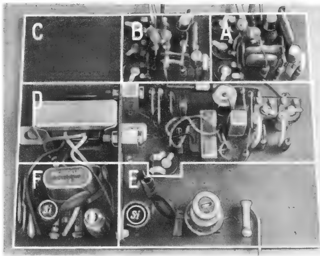
Bild 12. Die bestückte Grundplatte des Senders nach Bild 10. A = Tongenerator 1, B = Tongenerator 2, C = Platz für Tongenerator 3, D = Modulationsverstärker E = Hf-Endstufe, F = Hf-Oszillator
