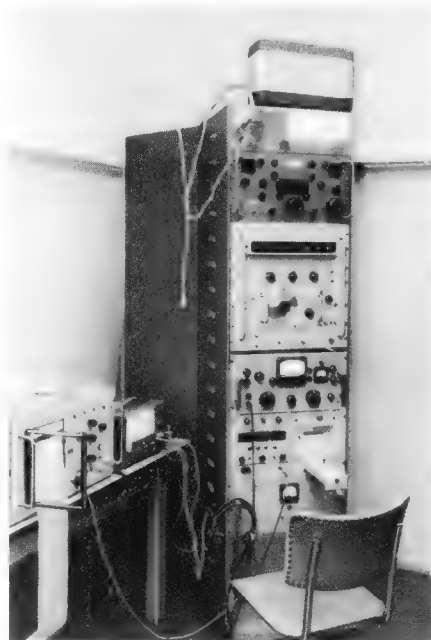
Bild 3. Empfangs- und Registrierplatz für Doppler-Effekt-Messungen
