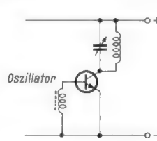
Bild 2. Als C-Verstärker geschalteter npn-Transistor
