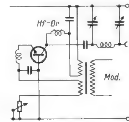
Bild 8. Emitterschaltung bei Emitterschaltung und geerdetem Kollektor
