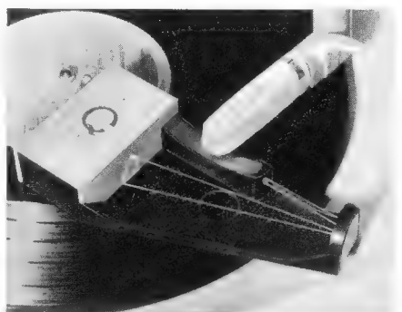
Bild 2. Der Nadelprüfer im Gebrauch; die Nadelspitze des Tonarmes wird in eine kleine Öffnung der sogenannten Prüfzelle eingetaucht, ihr vergrößertes Schattenbild entsteht auf der senkrechten weißen Fläche des Batteriegehäuses. Mit der Schraube an der Rückseite wird die Lampe eingeschaltet. Rechts der Spiegel, der den aus der Prüfzelle austretenden Lichtstrahl umlenkt
