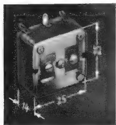
Bild 1. Abmessungen der Miniaturausführung eines Zweigang-Drehkondensators. Das Dielektrikum bildet eine auf die Statorplatten aufgespritzte Polyäthylenfolie
