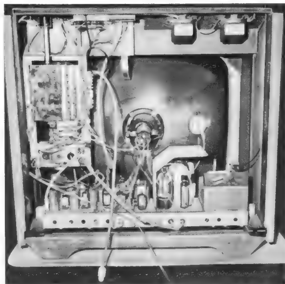
Bild 1. Neues französisches Fernsehgerät mit deutlich sich voneinander abhebendem Vorder- und Hinterteil
