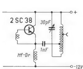
Bild 6. Endstufe eines Fernsteuerungssenders. Bei guter Anpassung erzielt man Leistungen bis zu 400 mW für Fernsteuerungssender
