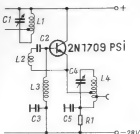
Bild 4. Endstufe in Emitterschaltung mit geerdetem Kollektor
